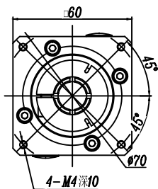
输入端 (INPUT)
