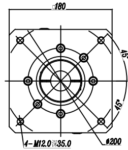
輸入端 (INPUT)
