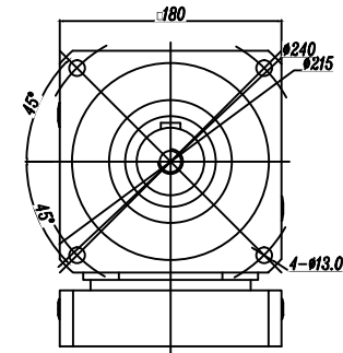
輸出端 (OUTPUT)
