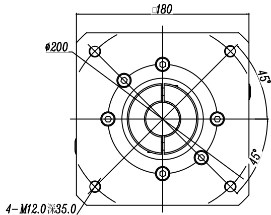
輸入端 (INPUT)
