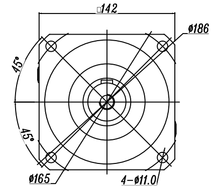
輸出端 (OUTPUT)
