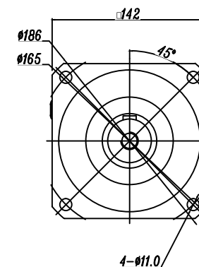
輸出端 (OUTPUT)
