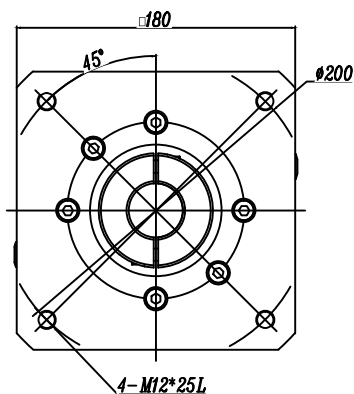
輸入端 (INPUT)
