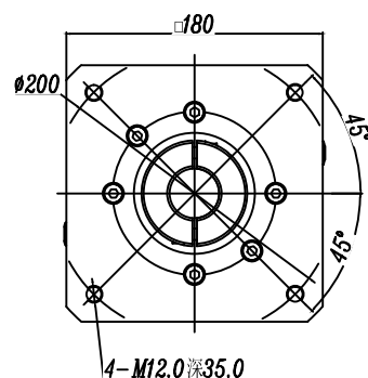
輸入端 (INPUT)
