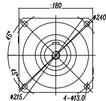
輸出端 (OUTPUT)
