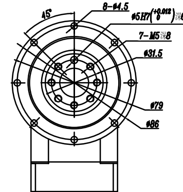
输出端 (OUTPUT)
