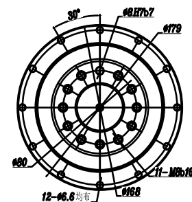
輸出端 (OUTPUT)
