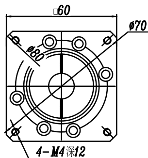
输入端 (INPUT)
