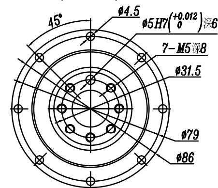
输出端 (OUTPUT)
