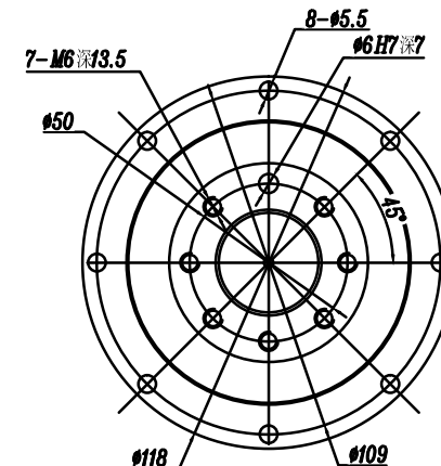
輸出端 (OUTPUT)
