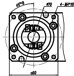
輸入端 (INPUT)
