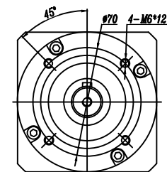
输出端 (OUTPUT)
