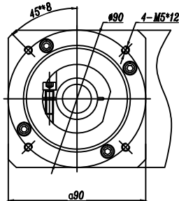
输入端 (INPUT)
