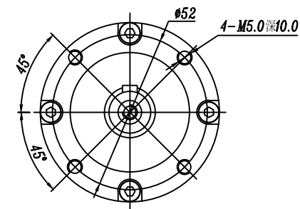
輸出端 (OUTPUT)
