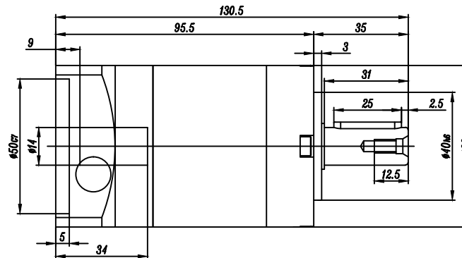
S2帶鍵:
