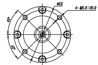
輸出端 (OUTPUT)
