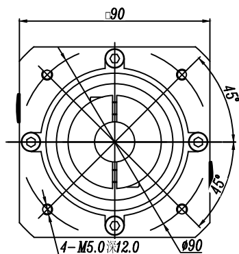
輸入端 (INPUT)
