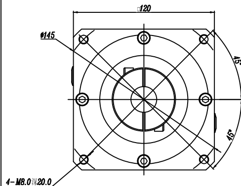
輸入端 (INPUT)
