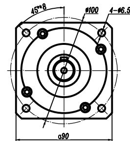
输出端 (OUTPUT)
