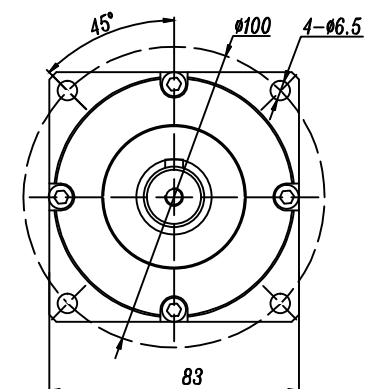
輸出端 (OUTPUT)
