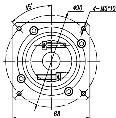
輸入端 (INPUT)
