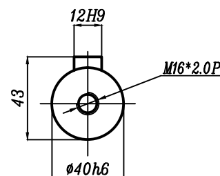
S2帶鍵:
