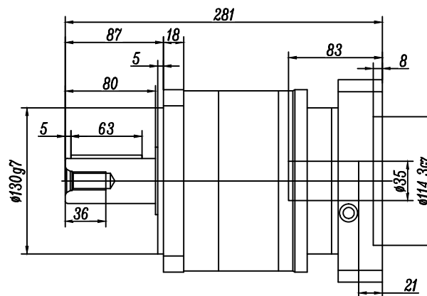
S2帶鍵:
