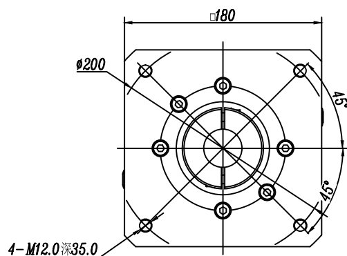
輸入端 (INPUT)
