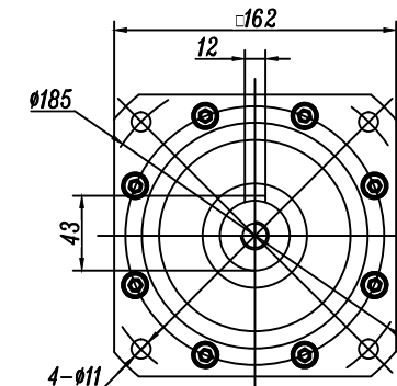
輸出端 (OUTPUT)
