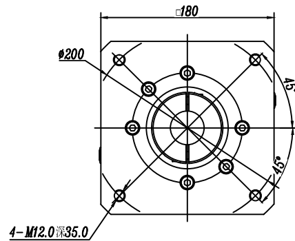
輸入端 (INPUT)
