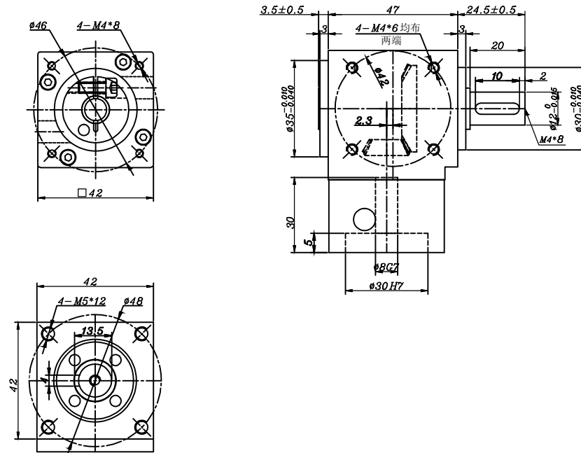
输入端 (INPUT)
