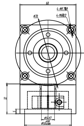
輸入端 (INPUT)
