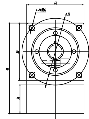
輸出端 (OUTPUT)
