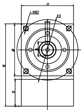
輸入端 (INPUT)
