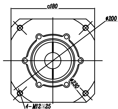
輸入端 (INPUT)
