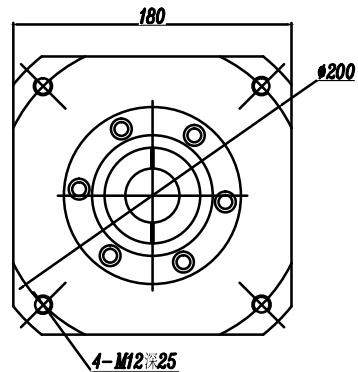
輸入端 (INPUT)
