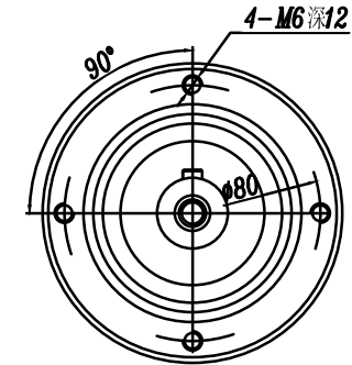
輸出端 (OUTPUT)
