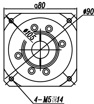
輸入端 (INPUT)
