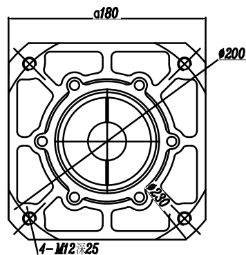
輸入端 (INPUT)
