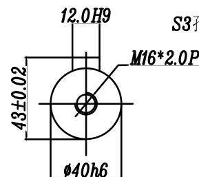
S2帶鍵:
