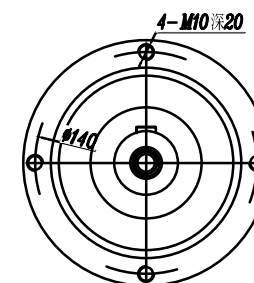
輸出端 (OUTPUT)
