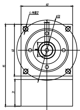
輸入端 (INPUT)
