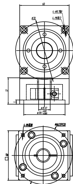
輸出端 (OUTPUT)
