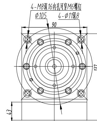
输出端 (OUTPUT)
