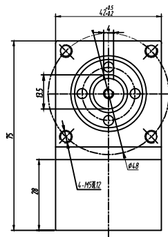
輸入端 (INPUT)
