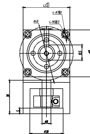
輸出端 (OUTPUT)
