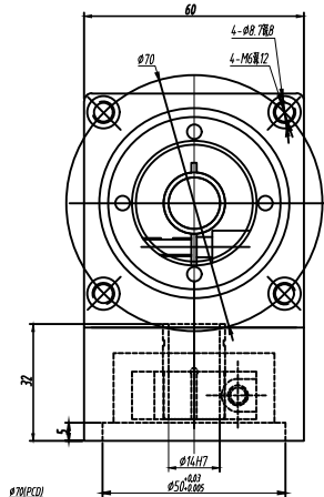
輸出端 (OUTPUT)
